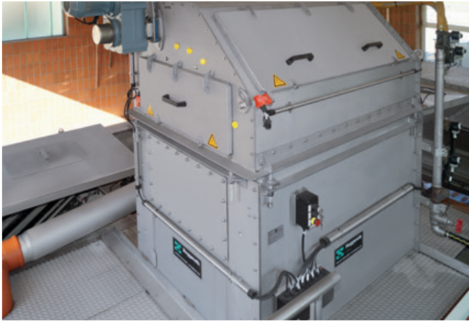
Noggerath® Siebbandrechen Centre-Flo™ CF
